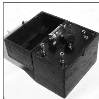
Krystalka RS s pevně zabudovaným detektorem. Vyrobila Radioslavia Praha cca 1925. Poslouchalo se na sluchátka. Foto: J. Jonášek
